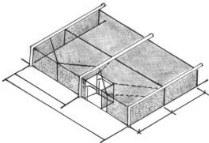
Figure 25 : Pépinière dans une petite serre libre d'insectes avec vanne à l'entrée (Rovero)
